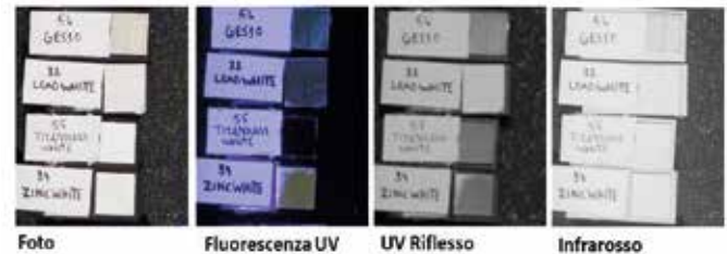
Fig. 5 - I quattro pigmenti bianchi di uso più comune stesi con gomma arabica e fotografati con quattro tecniche: fotografia normale, fluorescenza ultravioletta, ultravioletto riflesso, infrarosso. Dall'alto verso il basso i pigmenti sono: gesso, bianco di piombo, bianco di titanio, bianco di zinco.
